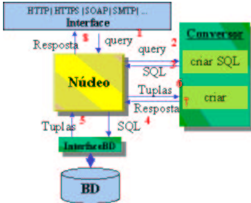
Figura 3.2: Arquitetura do Framework
