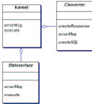
Figura 3.4: Diagrama de Classes do Framework
