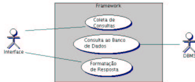
Figura 3.3: Diagrama de Use Case do Framework
