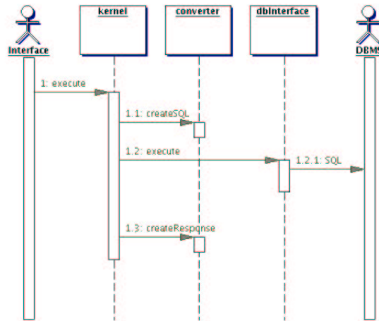
Figura 3.5: Diagrama de Sequência do Framework
